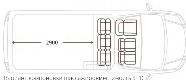
Вариант компоновки (пассажироместимость 5+1)
